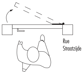
A1 Poussant droit Duwend rechts scharnierend
